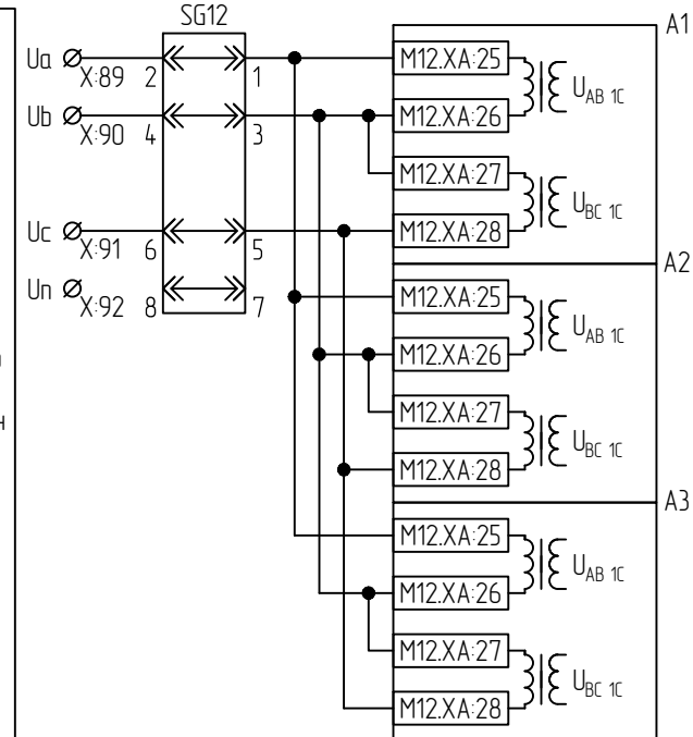
Цепи переменного напряжения 1 секции шир
