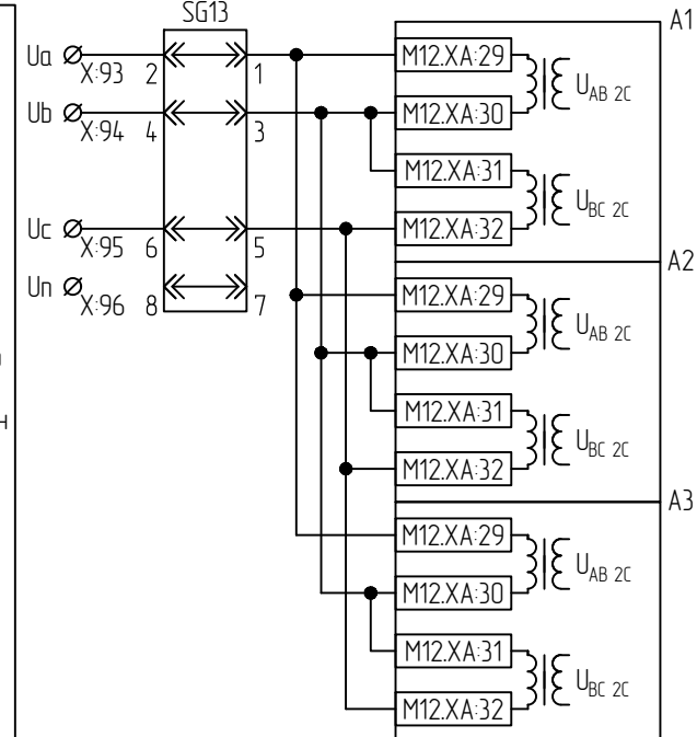
Цепи переменного напряжения 2 секции шп
